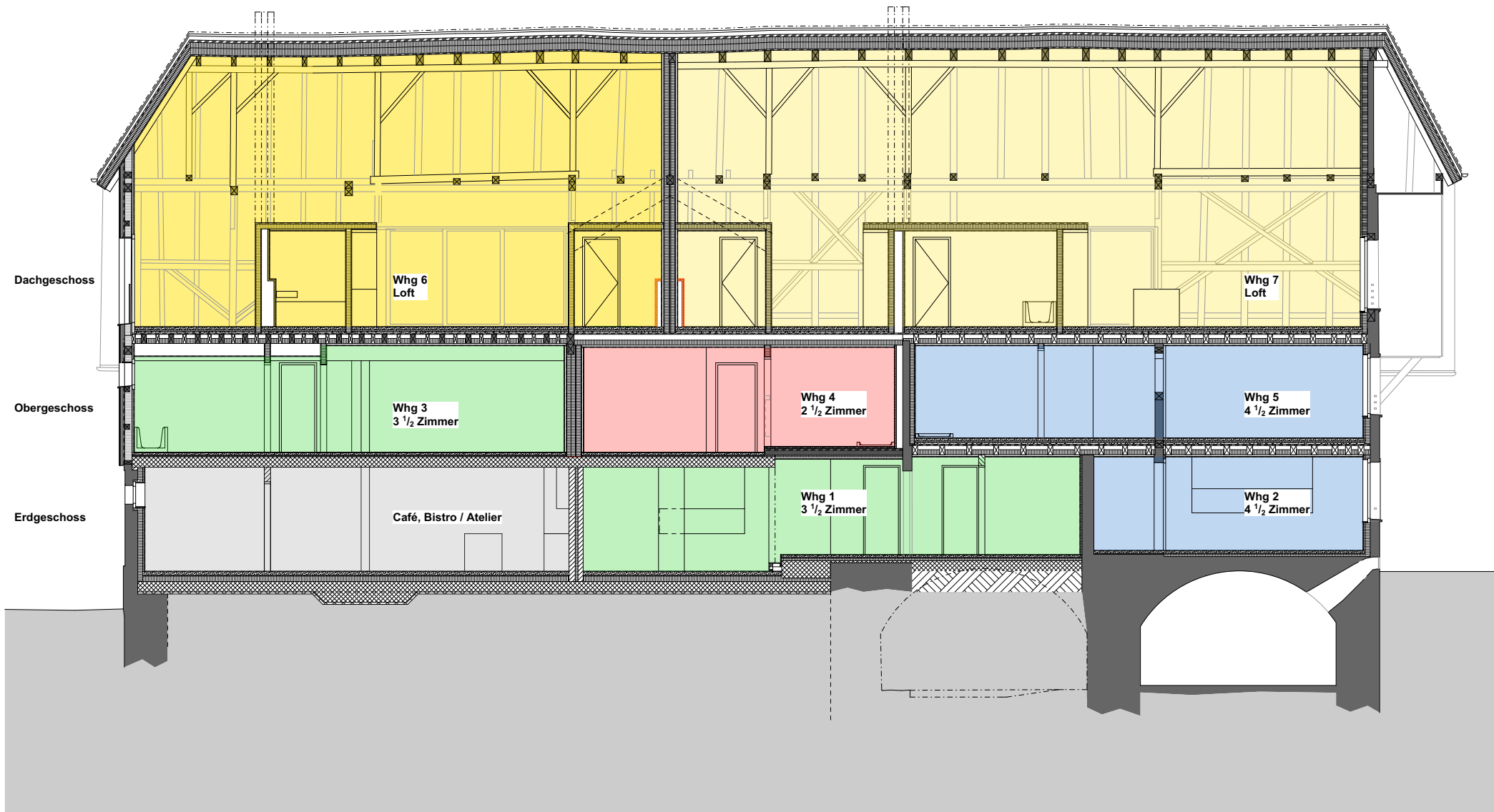
Schnitt Hirschen
